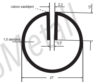
Mjerilu 1:1 Jedinica mjere: mm
