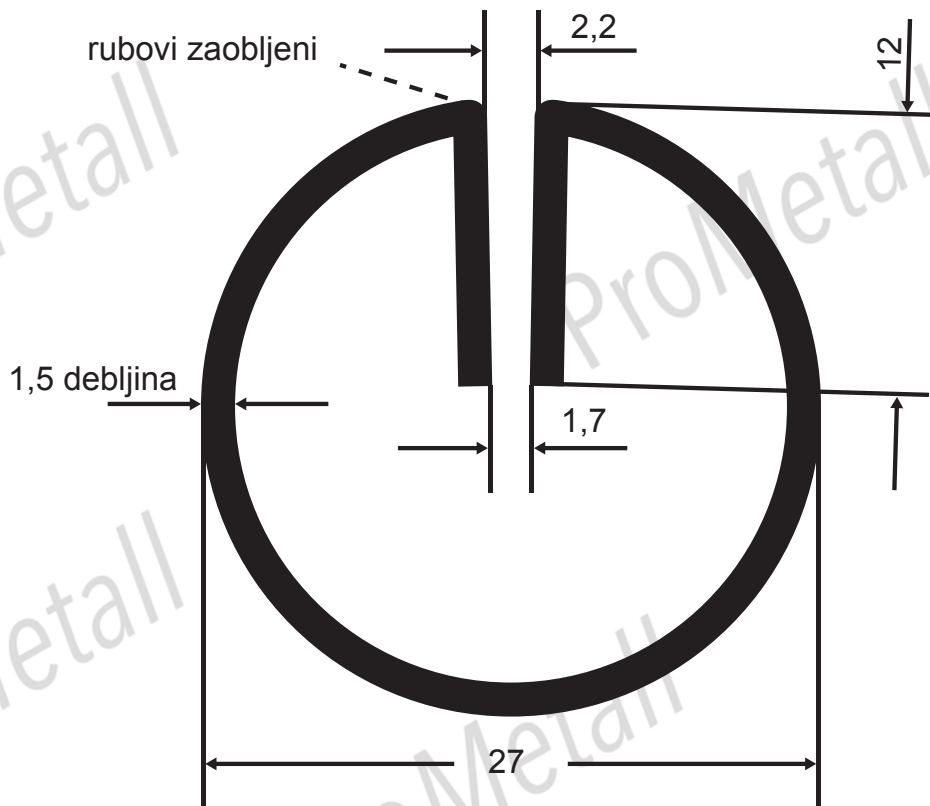
Mjerilu 3:1 Jedinica mjere: mm
